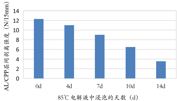
85°C 电解液中浸泡不同天数后层间剥离强度
